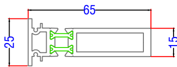
AL UK AW703 - Coupling Bar
