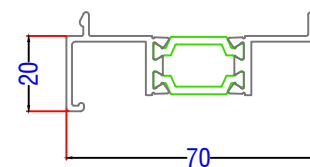
AL UK AW724 - Frame Extender
