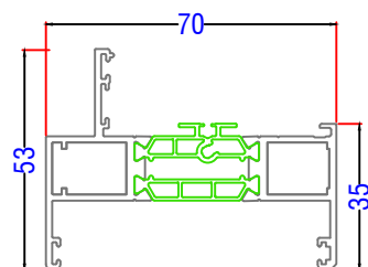
U44013- Outer Frame
